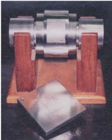
Moederplaat en molet
